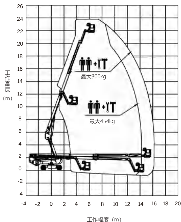
LT22JE-c 性能曲线图
